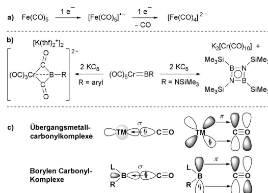
Abbildung 1. a) Ein- und Zweielektronenreduktion eines ÜM-Carbonylkomplexes; b) Reduktion von ÜM-Borylenkomplexen; c) Analogien der Orbitalwechselwirkungen zwischen CO und ÜM- bzw. Borylenfragmenten.
