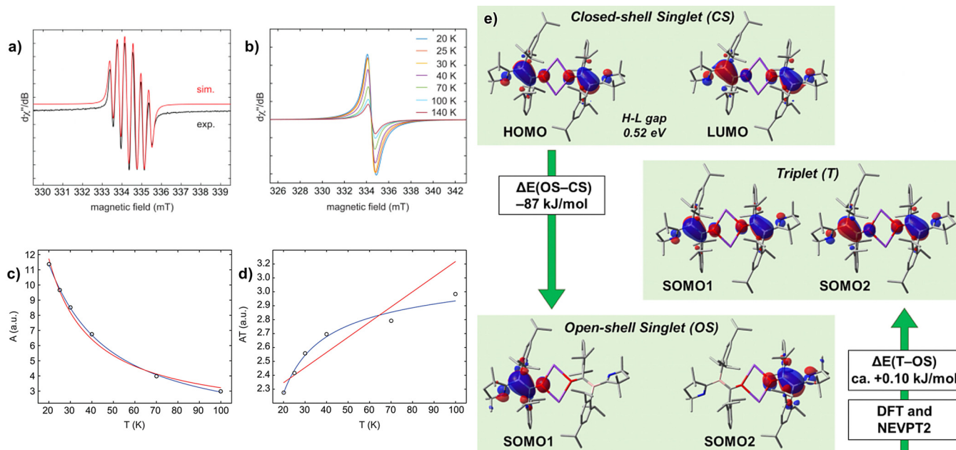
Abbildung 3. a) Experimentelles (schwarz) und simuliertes (rot) „continuous-wave X-band“-EPR-Spektrum von 3 in einer Toluol/THF-Mischung bei 270 K. Parameter der Simulation: g_{iso} = 2.0040 , a(^{11}\text{B}) = 11.7 MHz (4.2 G) und a(^{14}\text{N}) = 9.8 MHz (3.5 G). b) X-band-EPR-Spektrum von in KBr verdünntem 3 im Festkörper bei variabler Temperatur zwischen 20 und 140 K. Die aufgenommenen EPR-Spektren für reines Pulver sind im Wesentlichen identisch. c,d) Temperaturabhängigkeit der zweifachen integralen EPR-Intensität ( A ) von 3 . Kreise ( \circ ) repräsentieren die experimentellen Ergebnisse, die blaue Linie den Fit mit der Bleaney-Bowers-Formel und die rote Linie das Curie-Verhalten. e) Ausgewählte Grenzzustände von 3 im CS-Singulett-, Triplett- und OS-Singulett-Zustand mit den relevanten energetischen Unterschieden ( \text{kJ mol}^{-1} ), berechnet mittels DFT und NEVPT2.
