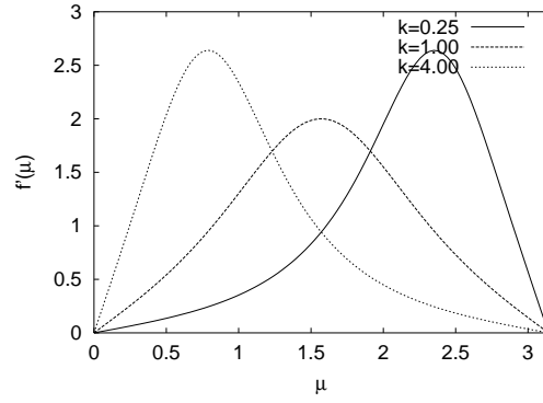
(d) f'(\mu) for B = 4
