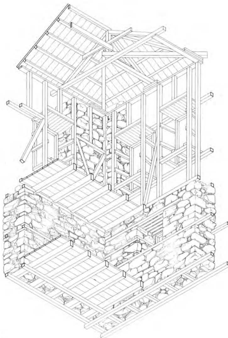
Σχήμα 6. Αξονομετρική τομή γωνίας κτιρίου όπου φαίνεται η σύνδεση του φέροντος οργανισμού της στέγης με τον ξύλινο σκελετό και τη λιθοδομή που αποτελούν τους εξωτερικούς τοίχους.
