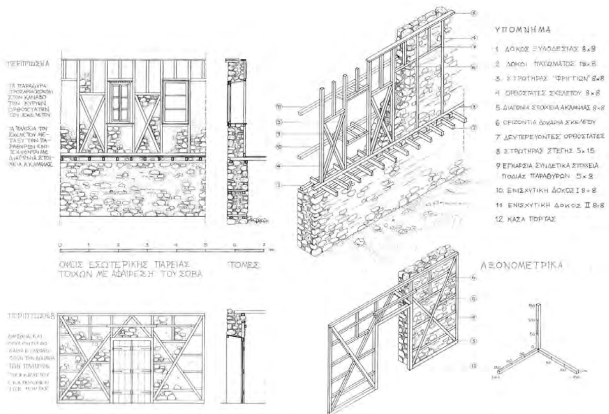
Σχήμα 3. Κατασκευαστικές λεπτομέρειες περιμετρικών τοίχων αποτελούμενων από διπλό φέροντα οργανισμό.
