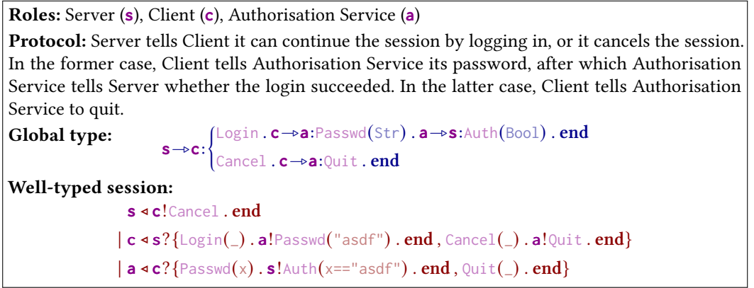
(a) OAuth2 Fragment
